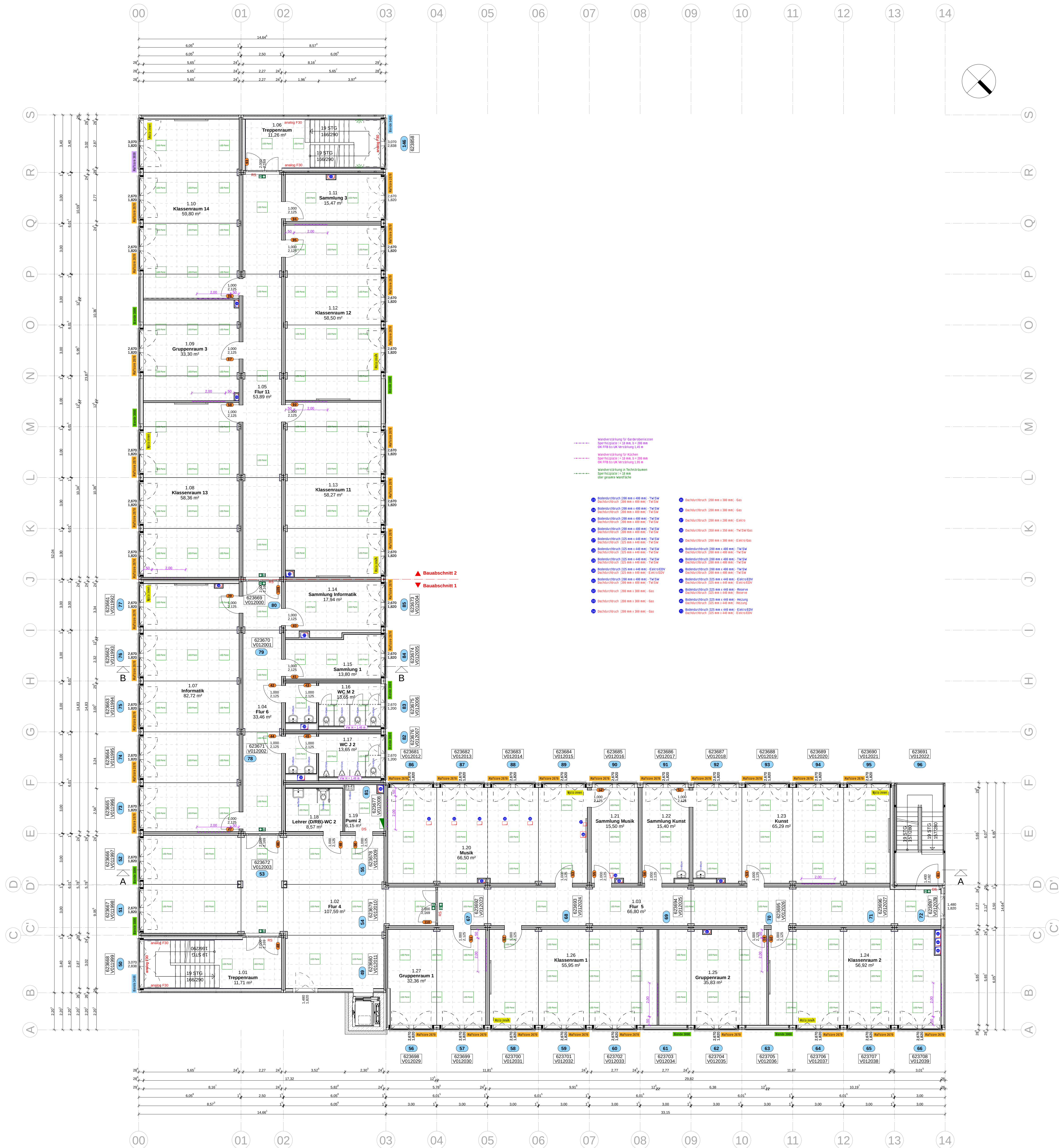
Grundriss 1. OG M 1:100
